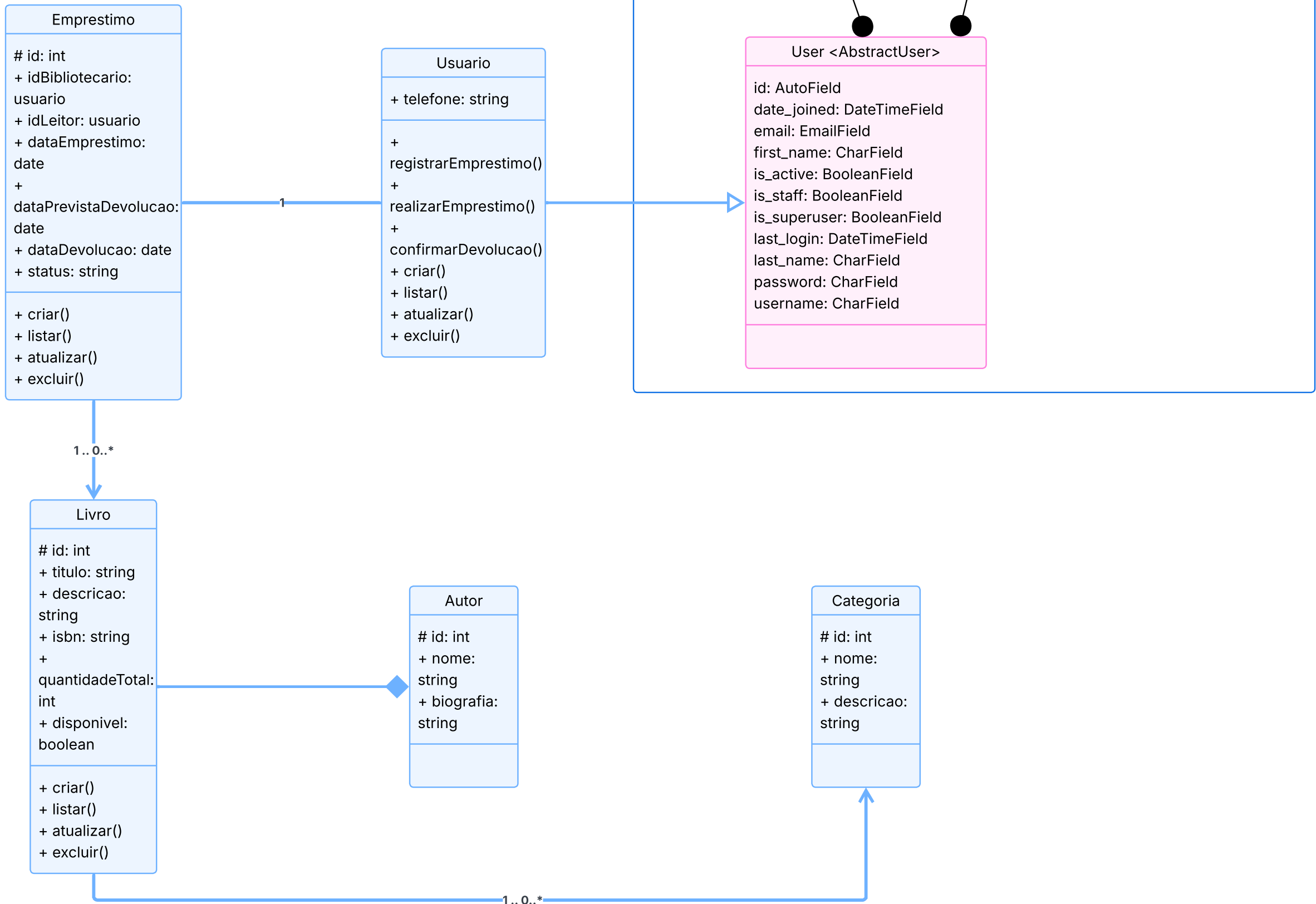
Diagrama de Classes UML - Biblioteca (Django)
